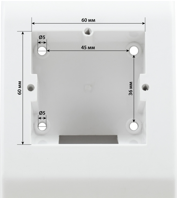
Проём и расположение отверстий
